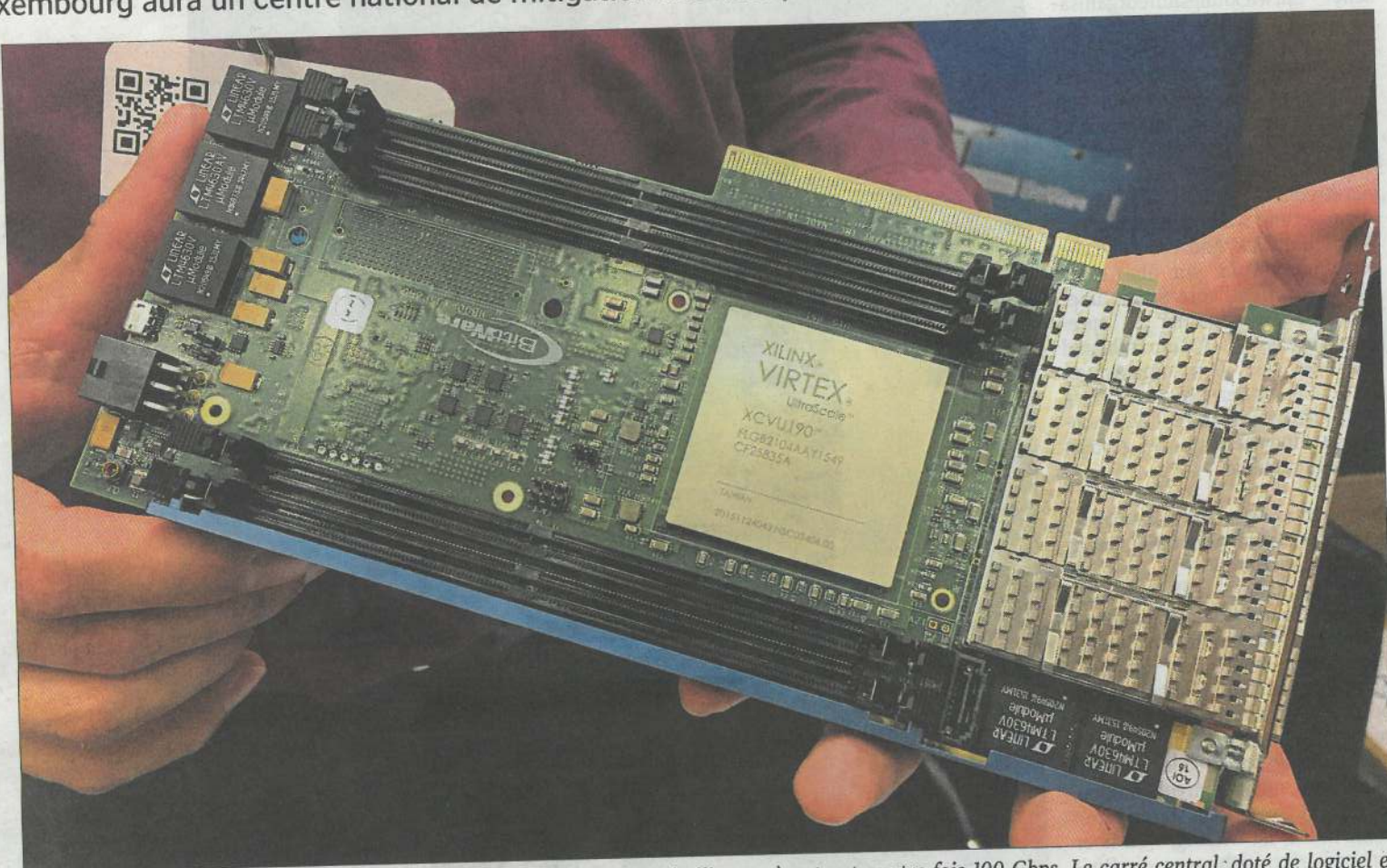
Un exemple d'«armoire de filtrage». A droite, les quatre barrettes métalliques où entrent quatre fois 100 Gbps. Le carré central, doté de logiciel et d'intelligence artificielle, détecte le trafic néfaste et le bloque. Le cœur du futur centre national de mitigation. (PHOTO: THIERRY LABRO)
